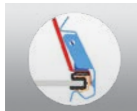
تأمین شرایط آببندی مطمئن با استفاده از نوار آببندی سیلیکونی و بستهای استنلس استیل Silicon gasket and stainless steel clips for long lasting high ingress protection
